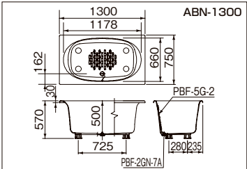
■ 写真はABN-1300です。 外寸法1,300×750×570 内寸法1,178×660×500 底面寸法950×525
